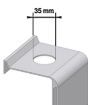
Montagebohrung 35 mm Tap hole 35 mm
