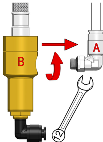
Winkelanschluss (A) mit 12er-Schlüssel lösen Disconnect the elbow fitting (A) with a 12 spanner
